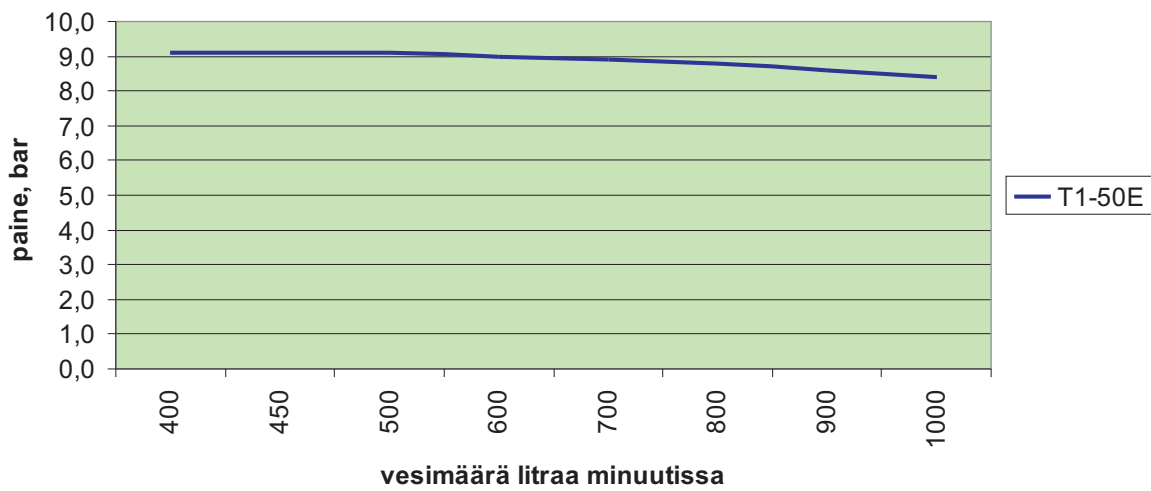
Rovatti T1-50E pumpun tiedot ulosoton pyörimisnopeudella 540 r/min
